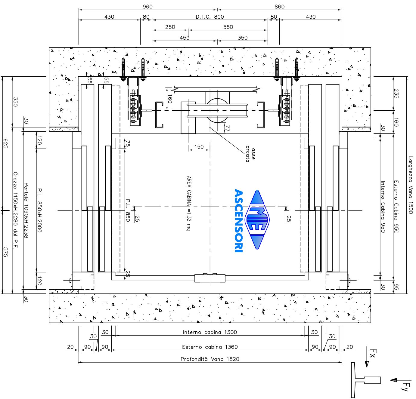
Pianta vano 480 kg
