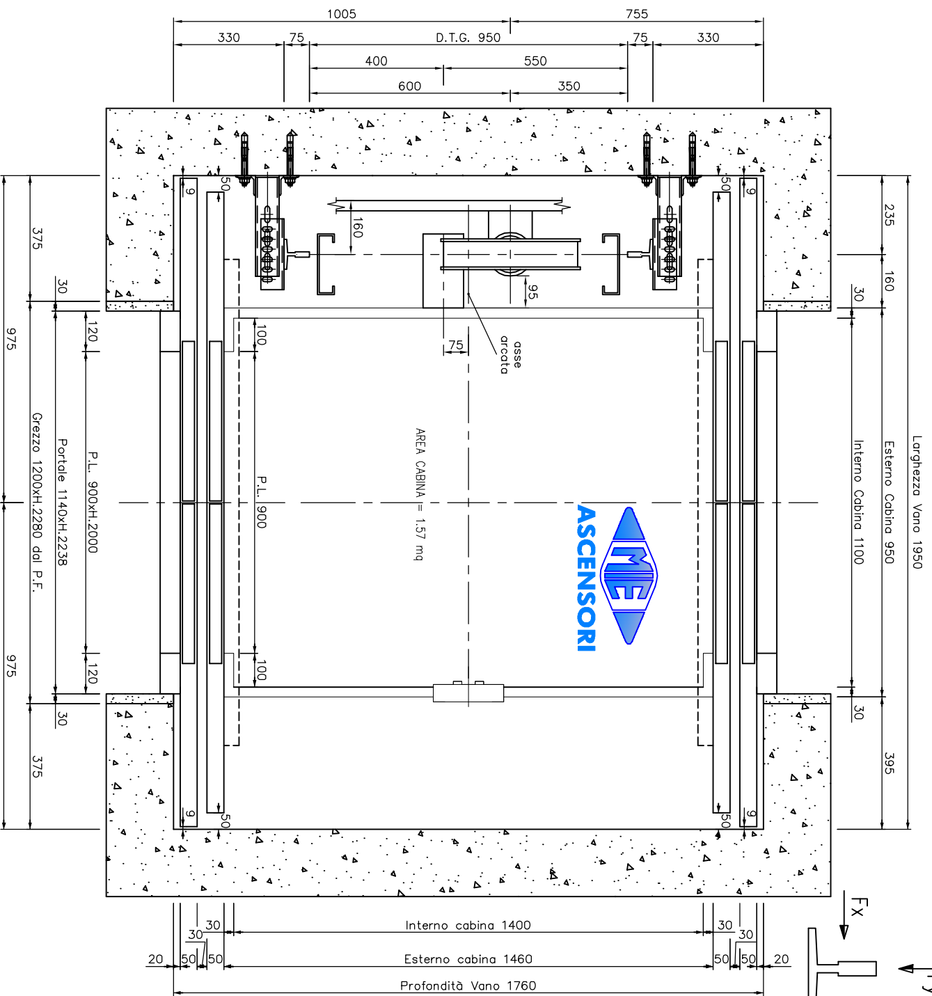
Pianta vano 630 kg
